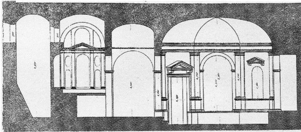
Spaccato e pianta della Camera Sepolcrale Petrucci sotto il Presbiterio della Chiesa di S. Domenico in Orvieto
