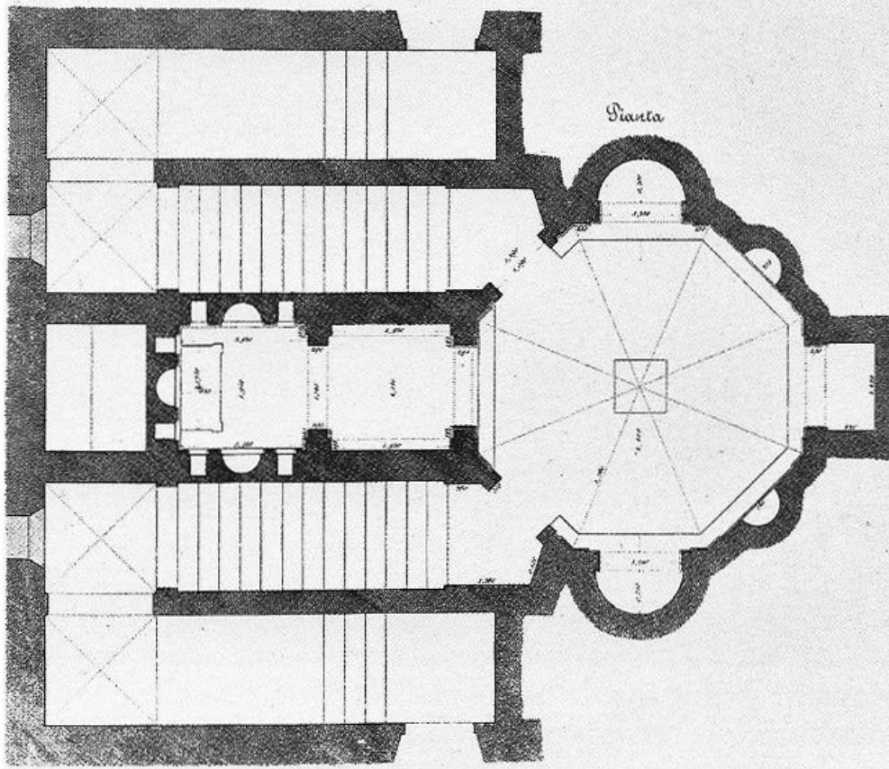
Spaccato e pianta della Camera Sepolcrale Petrucci sotto il Presbiterio della Chiesa di S. Domenico in Orvieto
