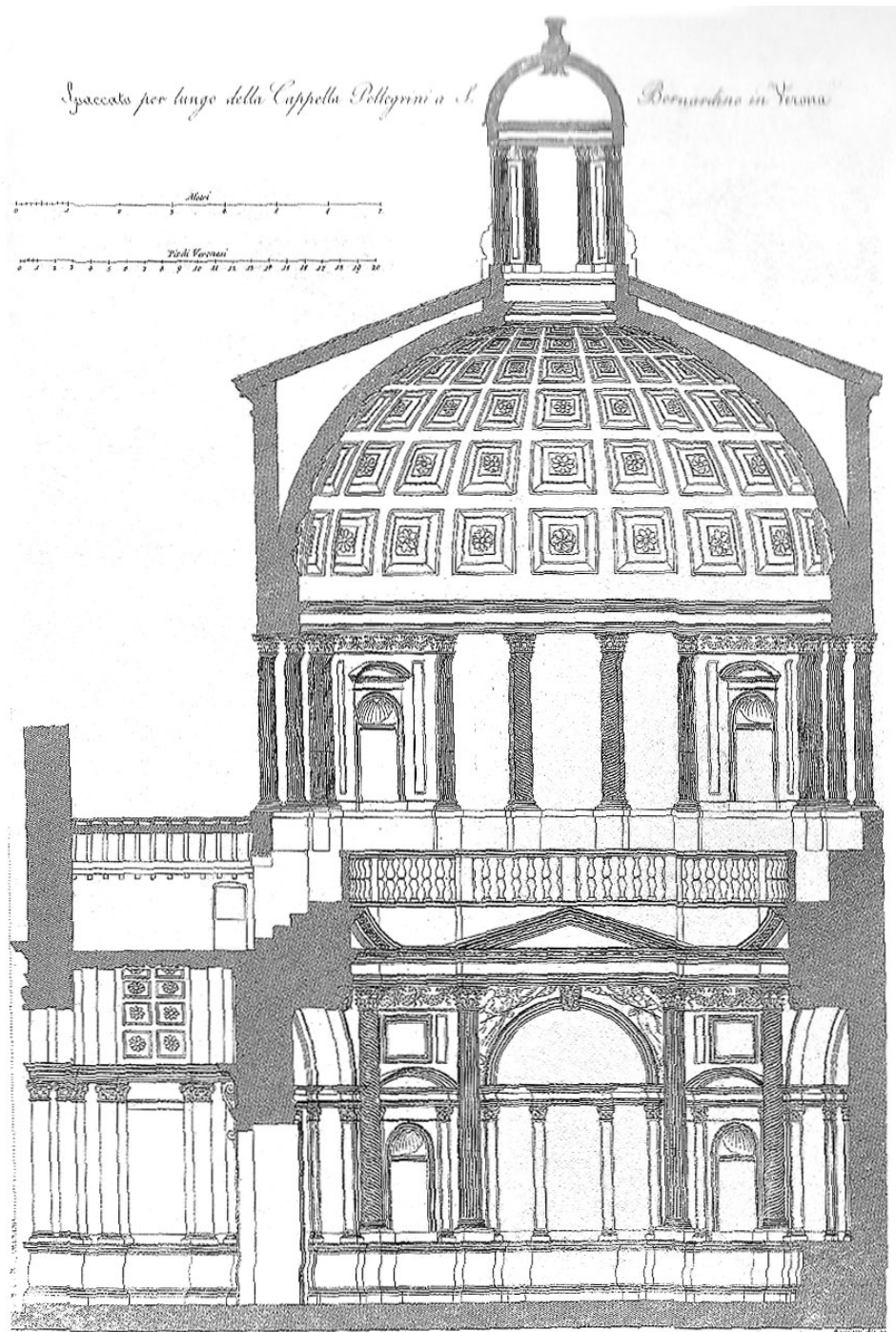
Cappella Pellegrini, Verona
